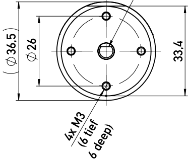
MB1 3601 Ø 6 mm Welle mit Abflachung Ø 6 mm Shaft
